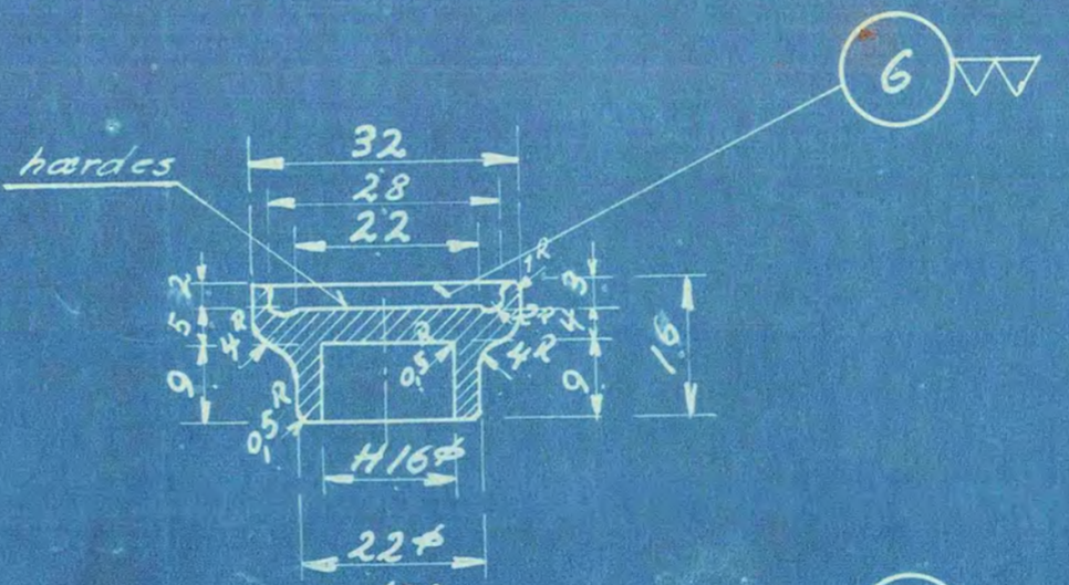
udbores og afdrejes henholdsvis efter Dorn og Pakring
