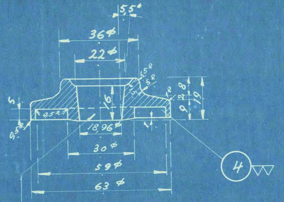
udbores og afdrejes henholdsvis efter Dorn og Pakring
